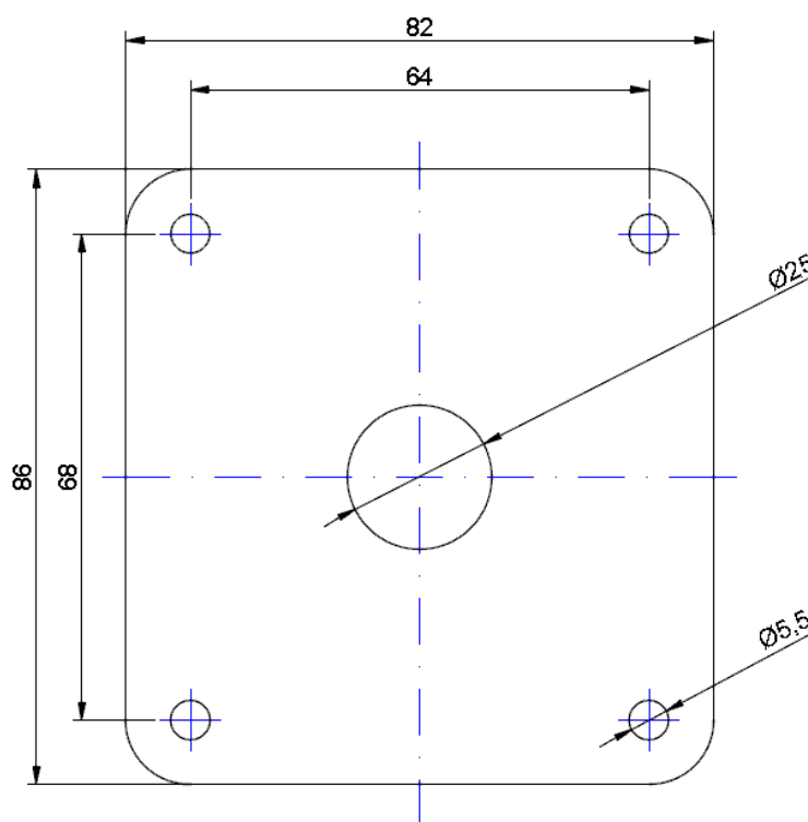
Рисунок 2. Присоединительные размеры ДУТ.
